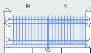
4 TRAVERSES 40x20 OU MÉPLAT 40x10 2 RANGÉES DE ROUNDS
