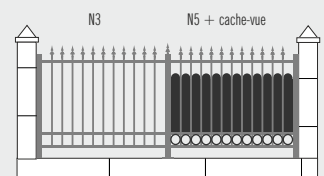
3 TRAVERSES SIMPLES 1 RANGÉE DE ROUNDS ET CACHE-VUE
